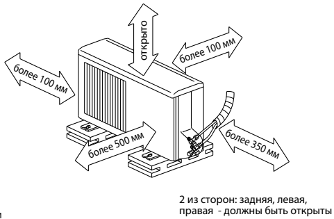
Пространство для установки
