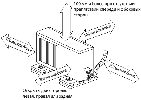
Пространство для установки
