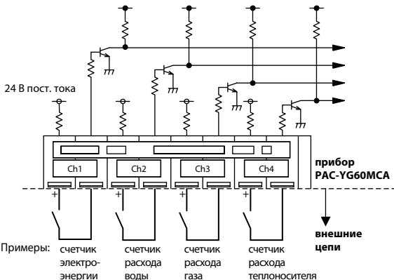
Подключение внешних цепей
