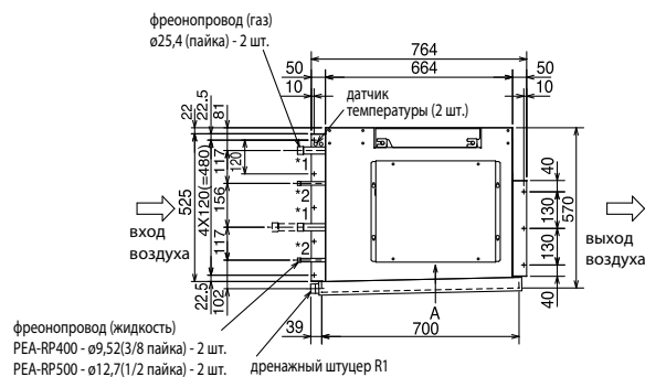
Вид слева РЕА-RP400/500GAQ
