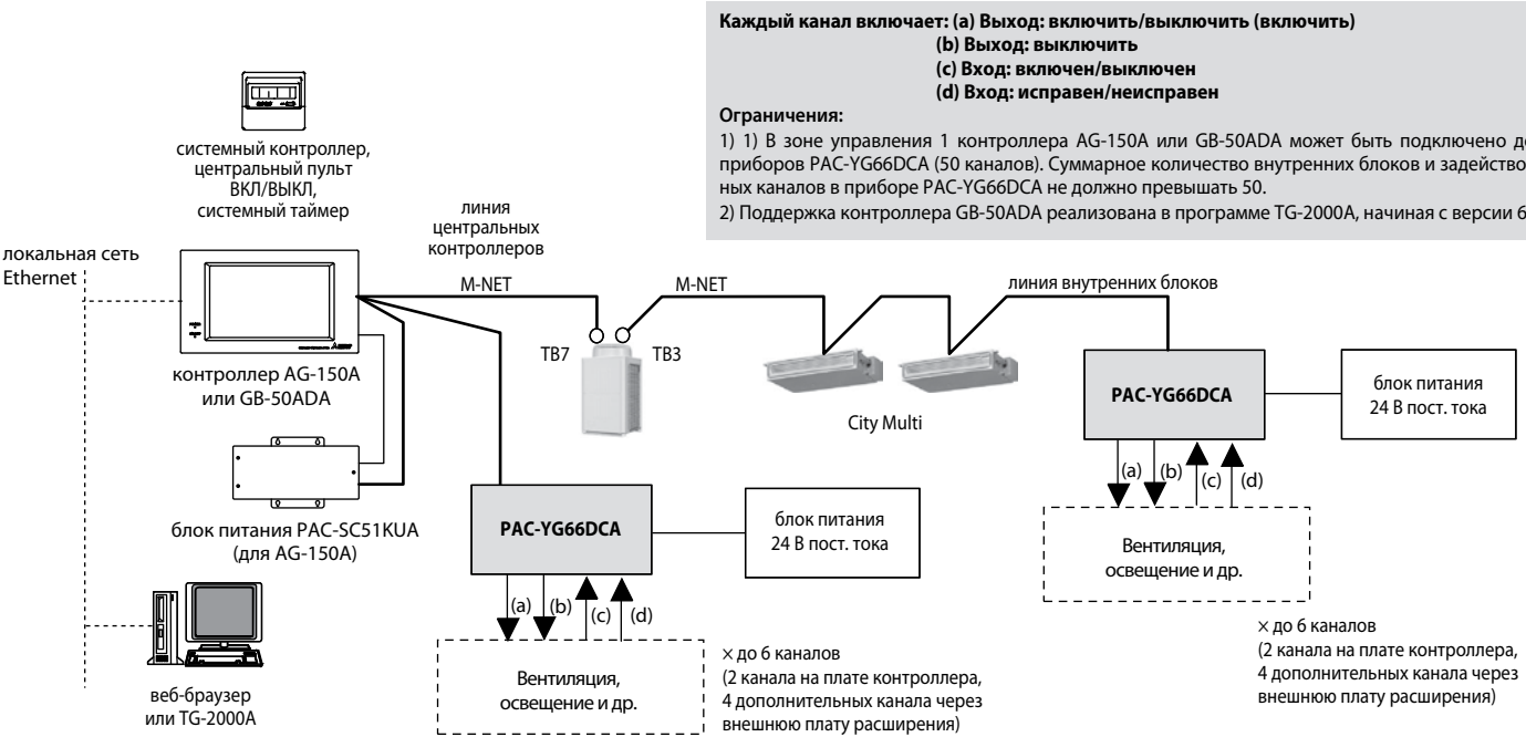
Подключение внешних цепей
