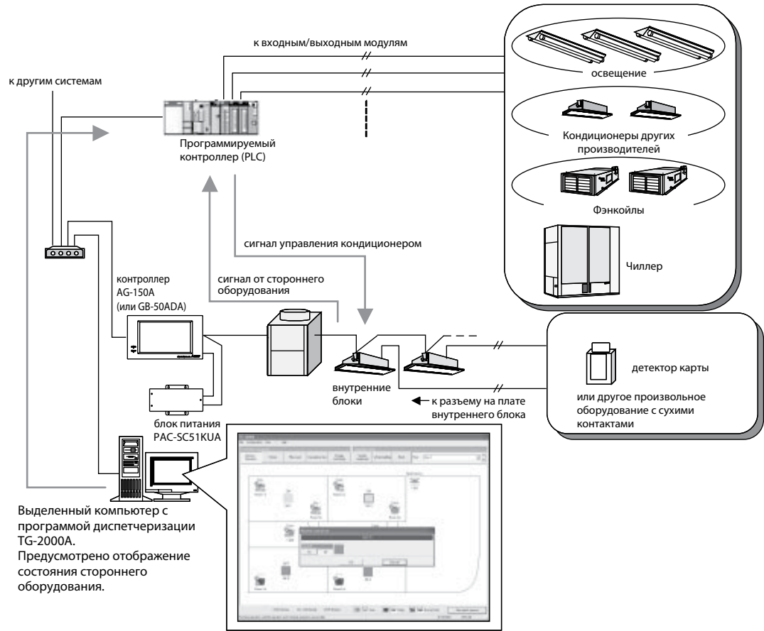
Состав аппаратно-программного комплекса
