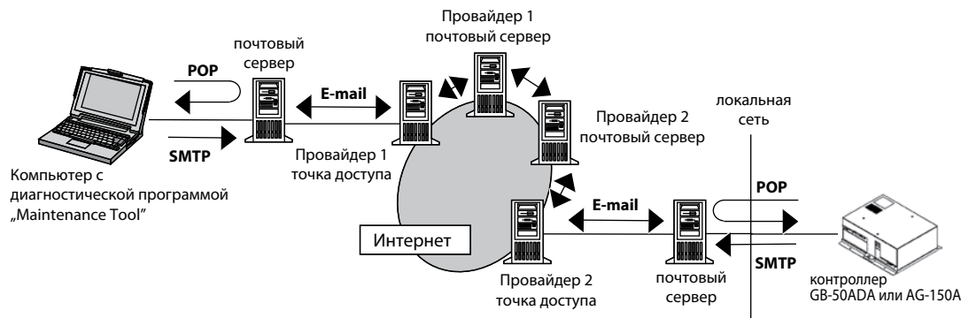
Состав аппаратно-программного комплекса
