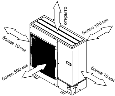
Пространство для установки
